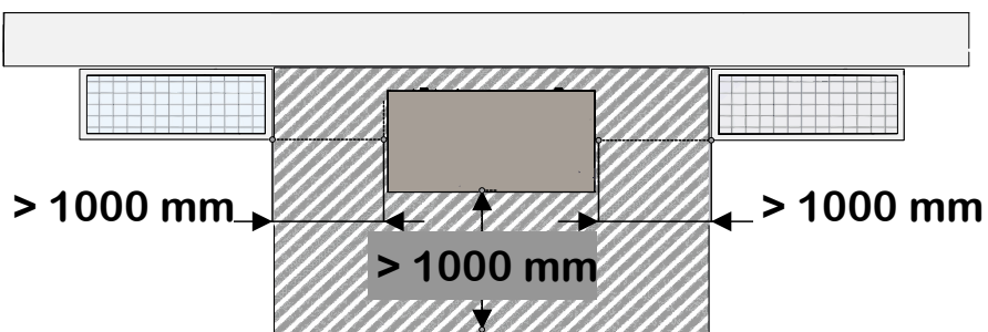
III. 2: Vista dall'alto dell'installazione su una parete chiusa
