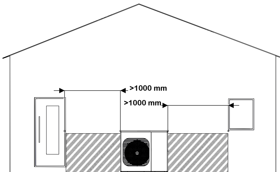
Ill. 1: Installazione su una parete chiusa
