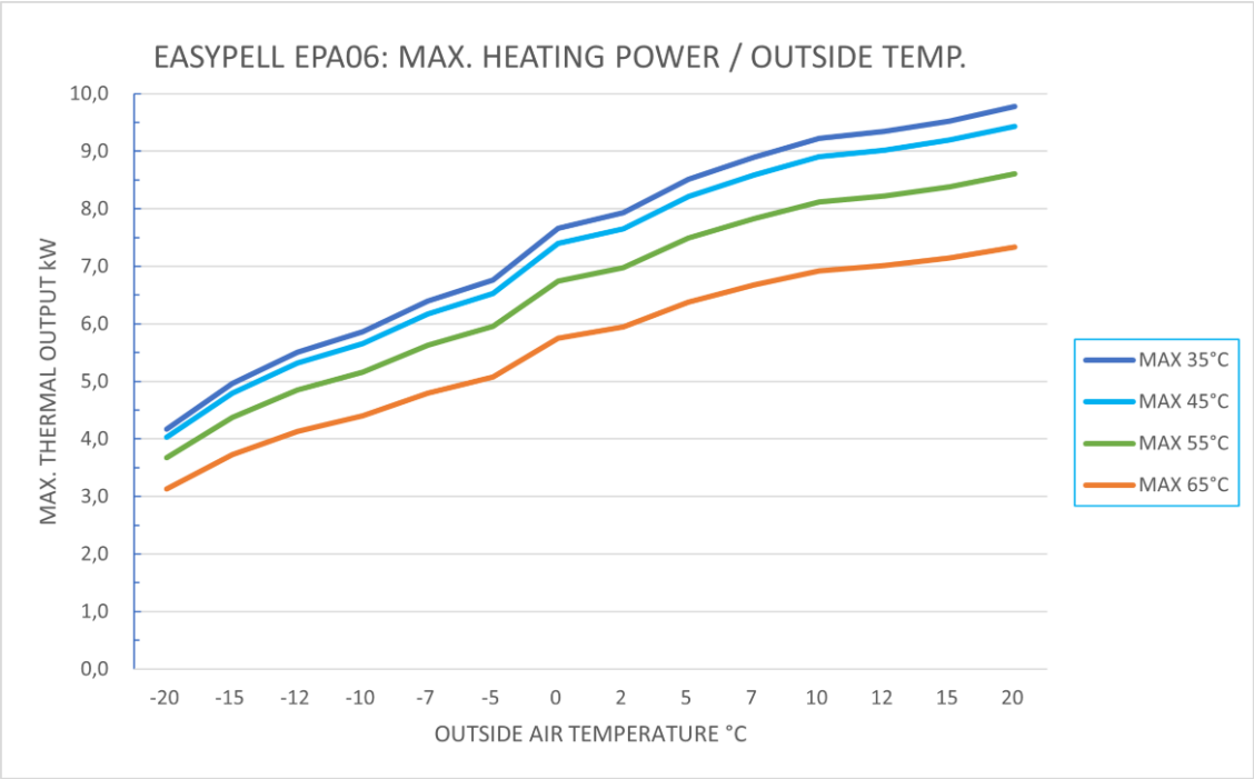
Curve di potenza EPA 06
